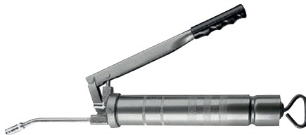
BOMBA DE ENGRASE MANUAL SAMOA 1431859 12SG. A palanca. Alto rendimiento. 500 cc. Válvula llenado 128 003 y acoplamiento rígido 710 214. Cartucho 400 g. Presión de entrega hasta: 500 bar. Caudal por embolada: 1,25 cc. Conexión salida de grasa: 1/8" NPT. 20'62 + IVA = 24'95
