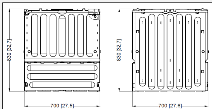
Compostadora Eco King 400L
