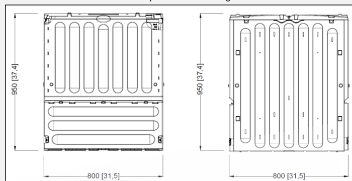
Compostadora Eco King 600L
